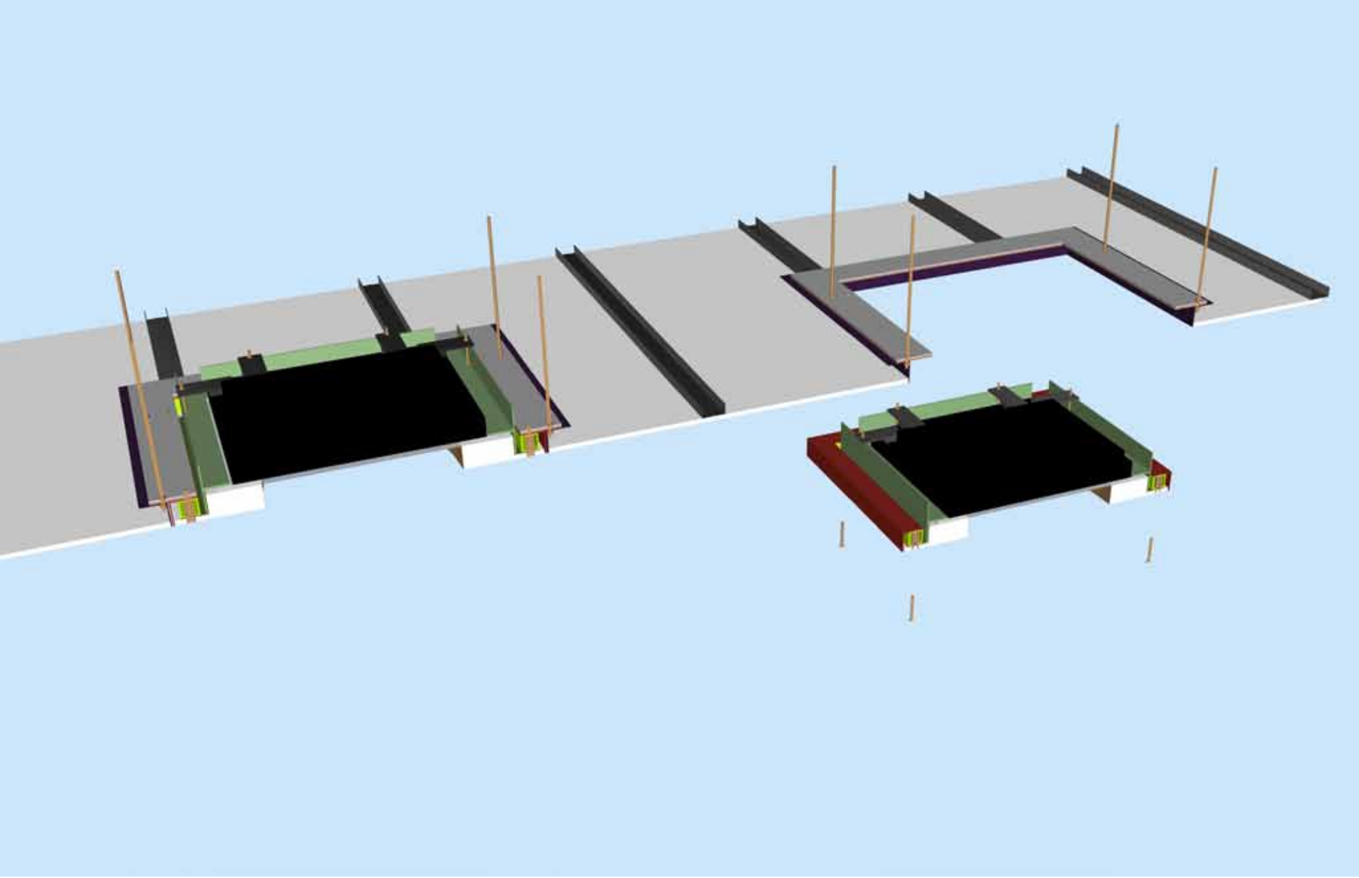
Rahmenmodul Decken-Montage Ansicht < von unten
