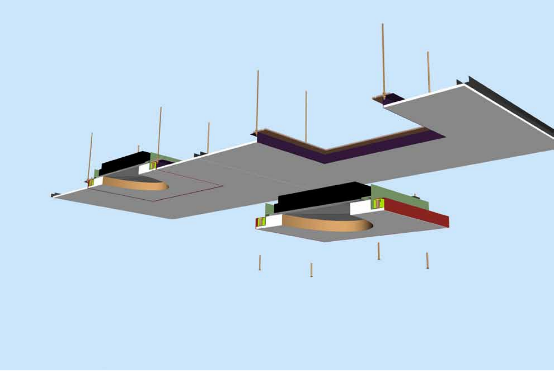
Rahmenmodul Decken-Montage Ansicht von oben >
