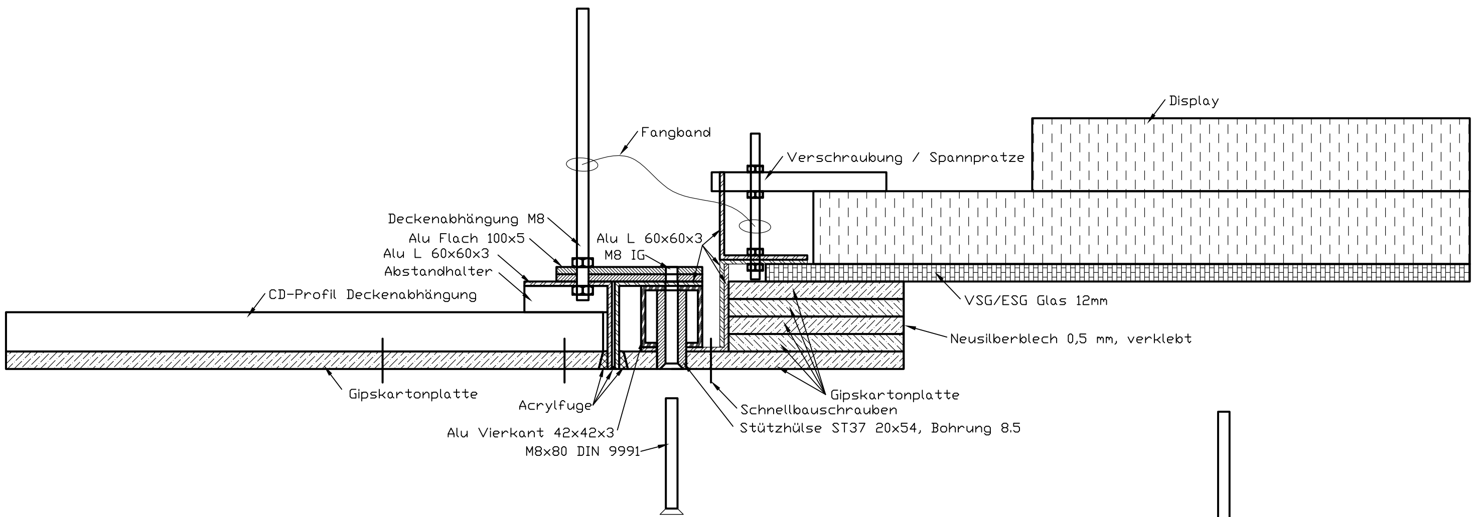
Aufbau eines Rahmenmoduls
